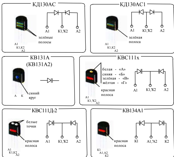
Рис. 5.3. Символьно-буквенная маркировка диодов
