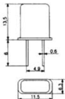
НС-49/S
