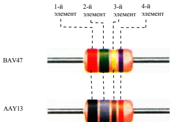
Рис. 5.6. Цветовая маркировка диодов по системе Pro Electron
