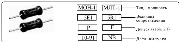
Рис. 1.2. Буквенно-цифровая маркировка выводных резисторов
