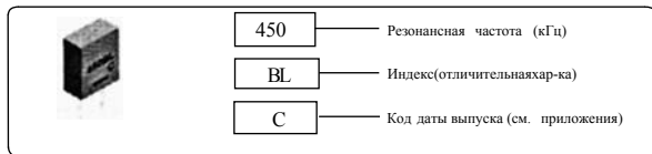
Рис. 4.2. Буквенно-цифровая маркировка керамических резонаторов
