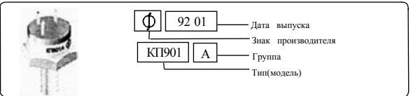
Рис. 6.6. Буквенно-цифровая маркировка отечественных транзисторов
