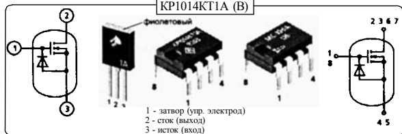
Рис. 7.5. Виды маркировки ключевых переключателей и стабилизаторов
