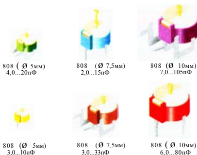
Рис. 2.13. Цветовая маркировка триммеров с плёночным диэлектриком (серия 808)
