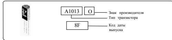
Рис. 6.3. Буквенно-цифровая маркировка транзисторов по системе «JIS»
