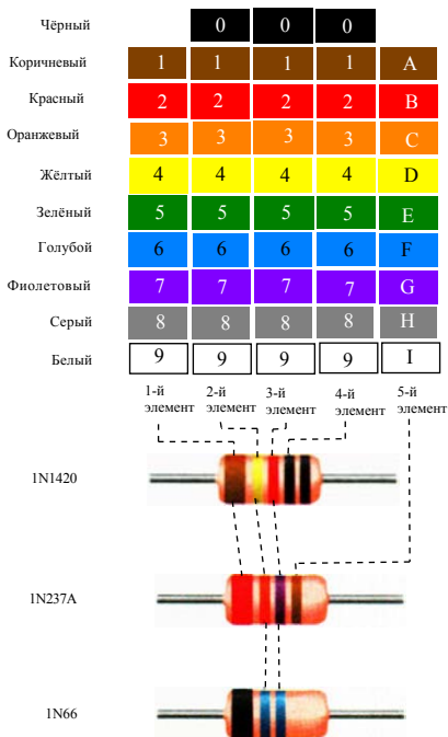
Рис. 5.5. Цветовая маркировка диодов по системе JEDEC
