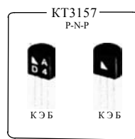
Рис. 6.25. Виды маркировки отечественных транзисторов
