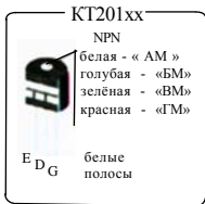
Рис. 6.10. Виды символично-цветовой маркировки отечественных транзисторов в корпусах КТ-26 (ТО-92)
