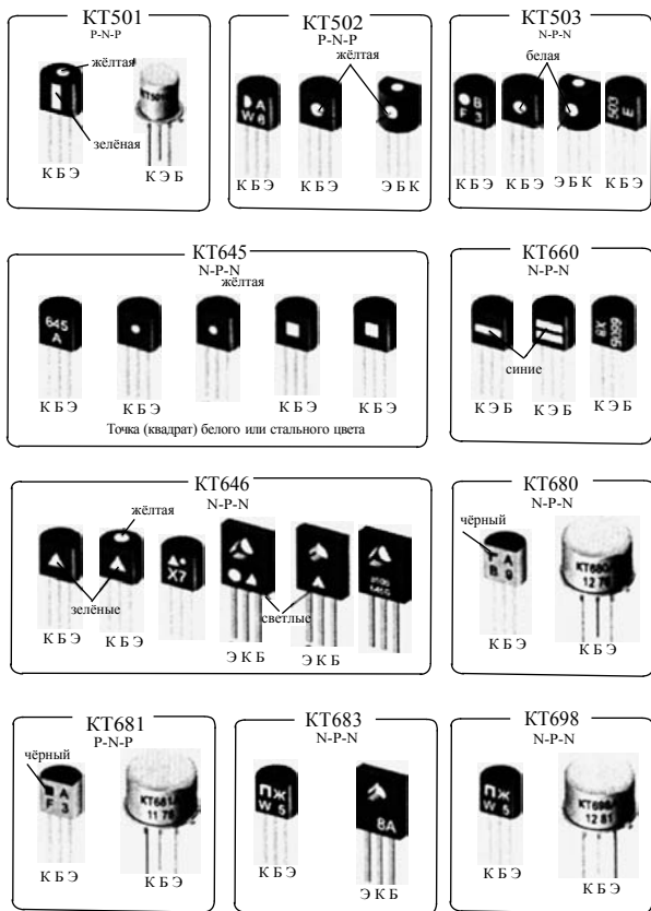
Рис. 6.26. Виды маркировки отечественных транзисторов в разных корпусах
