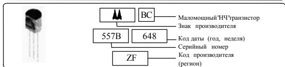
Рис. 6.2. Буквенно-цифровая маркировка транзисторов по системе «Pro Electron»
