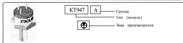
Рис. 6.5. Буквенно-цифровая маркировка отечественных транзисторов
