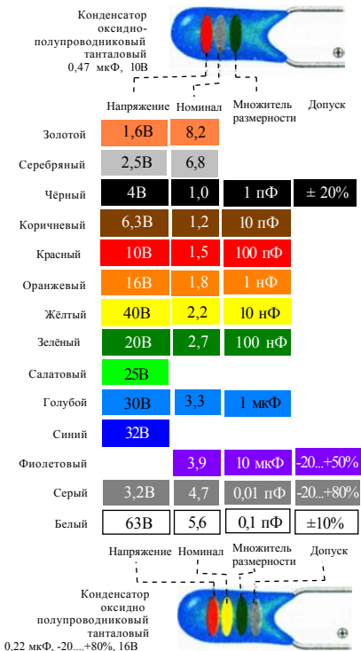
Рис. 2.12. Цветовая маркировка электролитических конденсаторов
