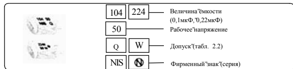
Рис. 2.3 Буквенно-цифровая маркировка конденсаторов
