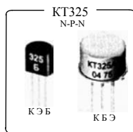
Рис. 6.23. Виды маркировки отечественных транзисторов
