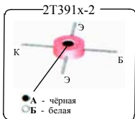
Рис. 6.16. Маркировка транзисторов в корпусах SOT-346 (SC59) и КТ-21
