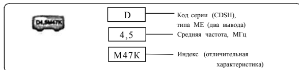
Рис. 4.6. Маркировка дискриминаторных фильтров
